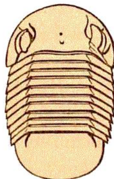
Illænus Barriensis.
