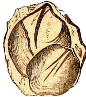
Pentamerus oblongus.
