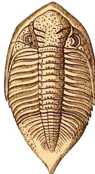
Phacops caudatus.
