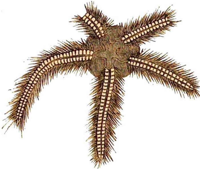
Protaster Miltoni.
