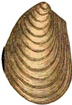
Inoceramus mytiloides.
