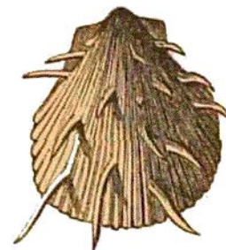
Lima spinosa.
