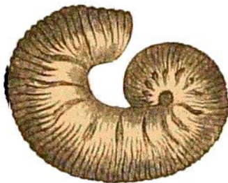
Scaphites æqualis.
