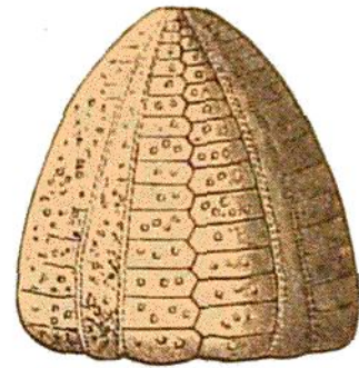
Echinoconus albo-galerus.
