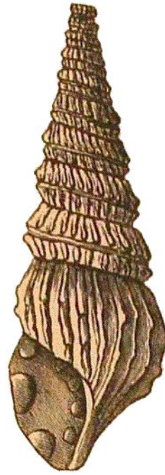
Turrilites costatus.
