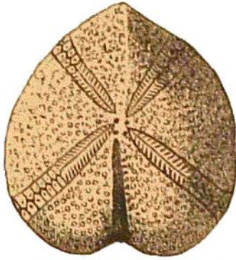
Micraster cor-anguinum.
