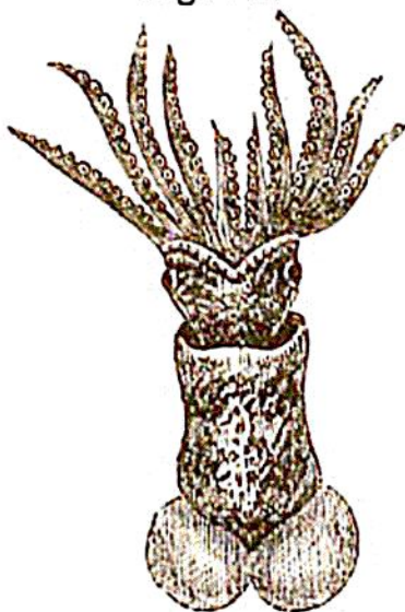
Loligo cardioptera.
