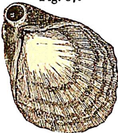
Terebratula.
