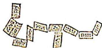
Bacillaria multipunctata.
