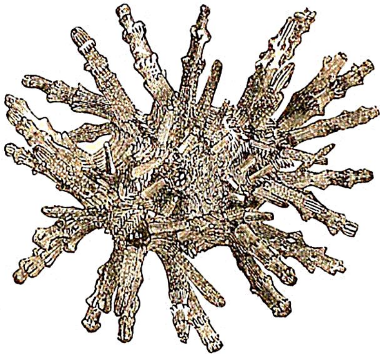
Echinus.
