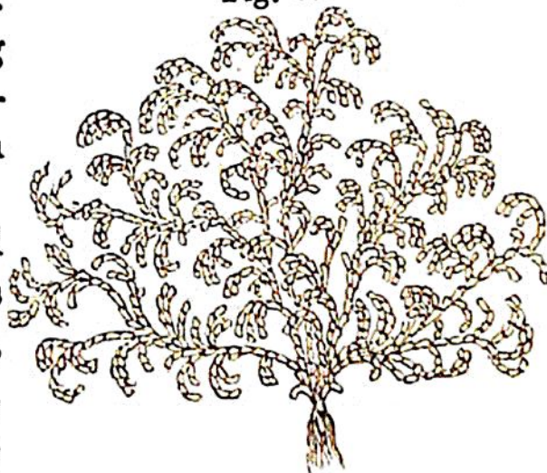
Cellaria cirrata.
