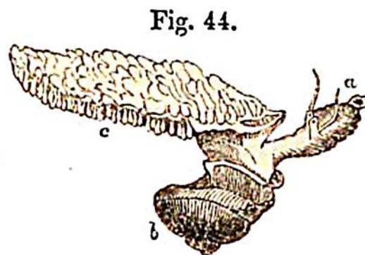
Ianthina.
