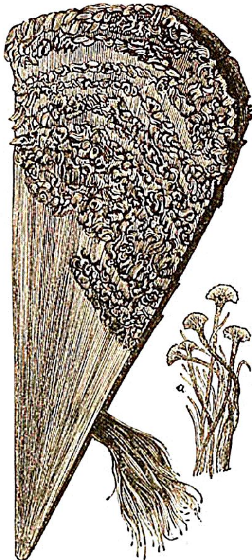
Pinna muricata.
