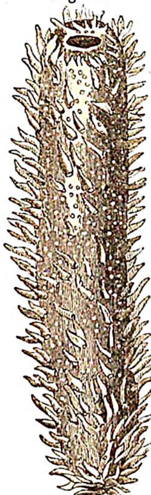
Pyrosoma giganteum.
