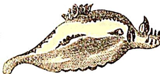
Polycera capensis.
