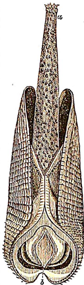
Pholus dactylus.
