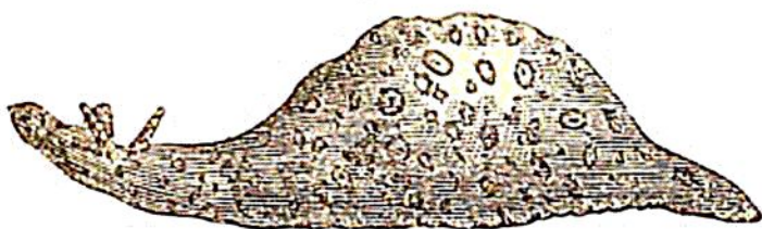
Laplysia.
