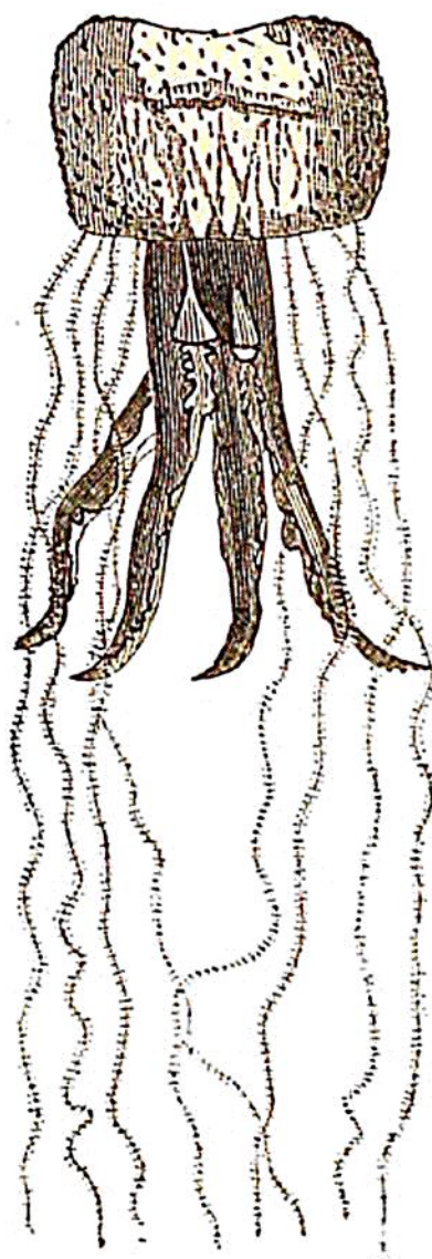
Rhizostoma.
