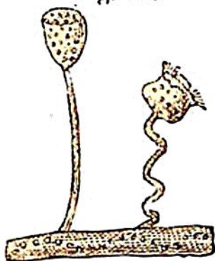
Vorticella cothurnata.
