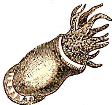
Spirula australis.
