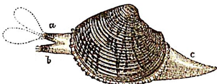
Venus Gallina.
