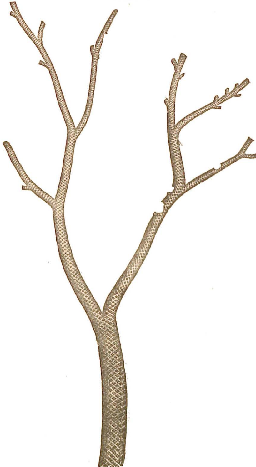
LEPIDODENDRON STERNBERGII.
