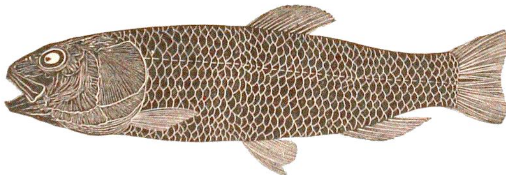
TELEOST. — Osmeroides Lewesiensis ( \times \frac{1}{2} ).
